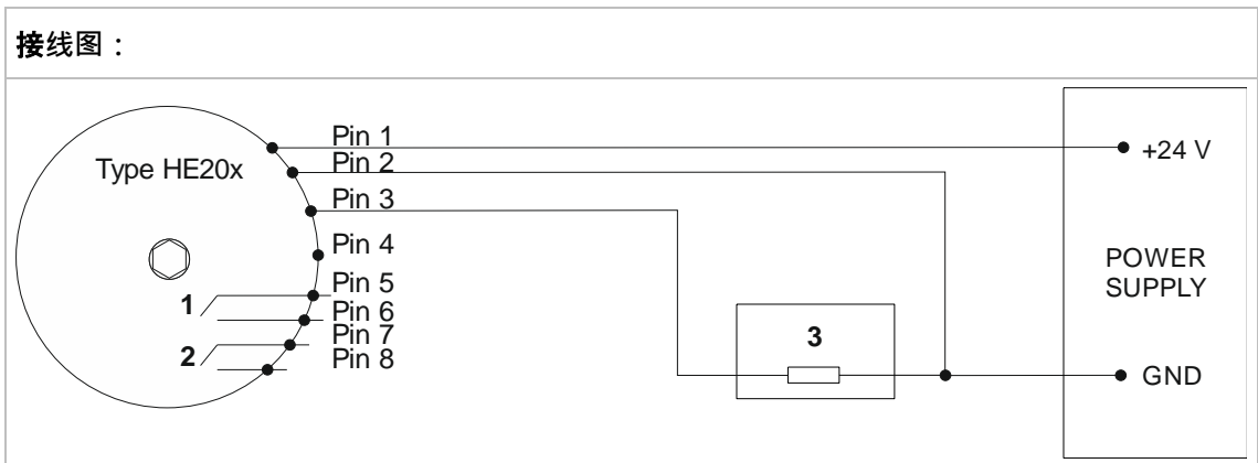
图 7：接线图
