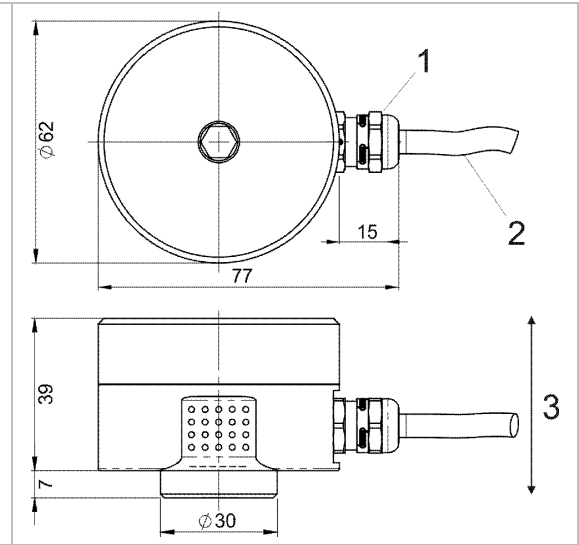
图 5：带集成式电缆的外壳
