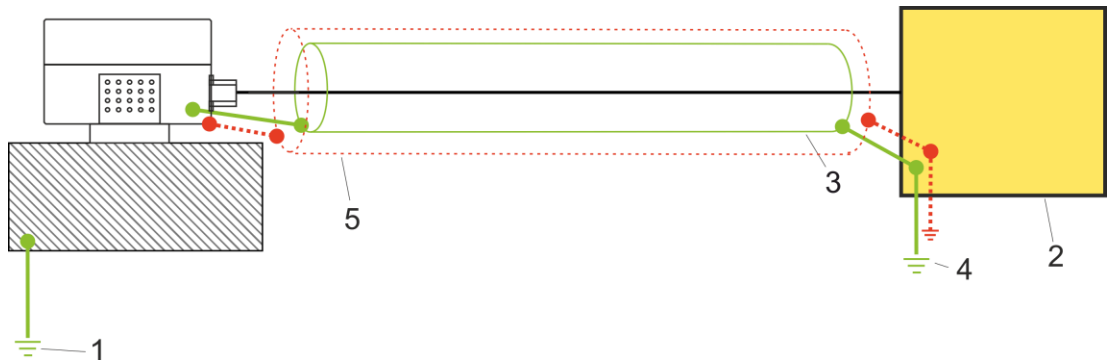
图 9：接地方案 HE200
