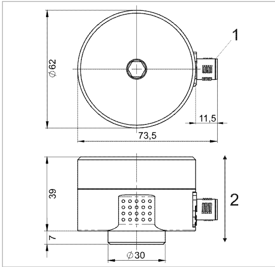
图 4：带 M12 插塞连接器的外壳
